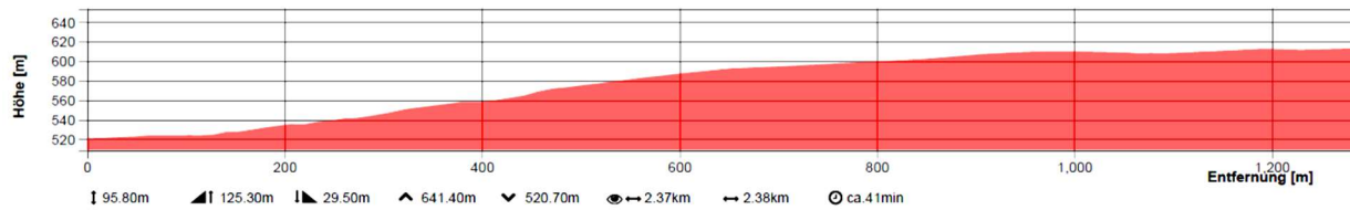
Profil Ottoberg - Aussichtsrestaurant Thurberg (11.45 - 12.35)
